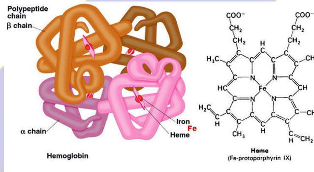
Gambar 2.1 Struktur Hemoglobin
